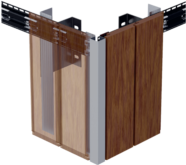
Flachschiene auf L-Profil an Wandhalter mit vertikalen Holzprofilen
