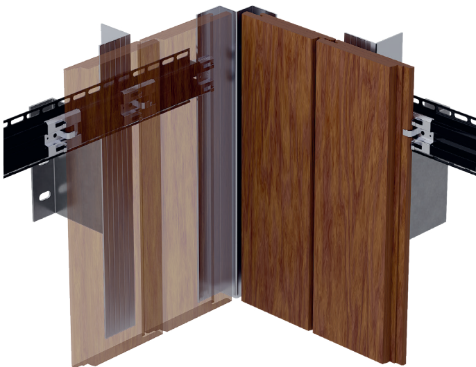
Flachschiene auf L-Profil an Wandhalter mit vertikalen Holzprofilen
