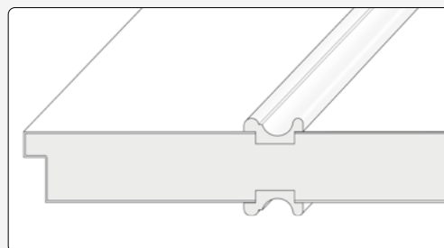
Türblatt mit eingefrästen und eingesetzten Leisten.
