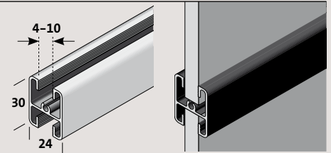
Füllungsteilerder Alusteg
