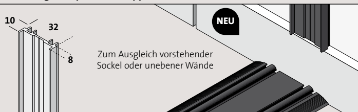
Wandausgleichsprofil, aufdoppelbar
