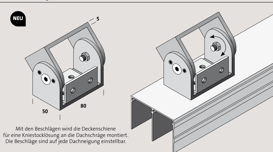
Kniestockbeschlag, Aluminium
