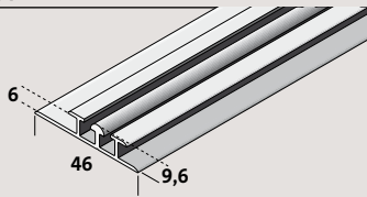
Einspurige Teppich-Bodenschiene
