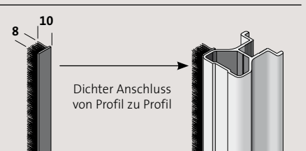
Staubbürste
