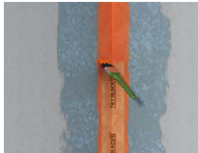
Abb. 2+3: fermacell™ Dichtband in die zuvor aufgetragene, noch feuchte fermacell™ Flüssigfolie drücken und direkt mit Flüssigfolie überstreichen – Trocknungszeit mind. 1 Stunde
