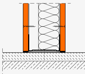
Trennwand auf Verbundestrich ( R_{L,w,R} ) = 38 bzw. 44 dB*
