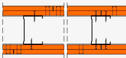
Montagewand mit fermacell® Gipsfaserplatten ohne Hohlraumdämmung als Einfachständerwand, doppellagig bekleidet. Äußere Plattenlagen in 1./untere Plattenlagen geklammert
