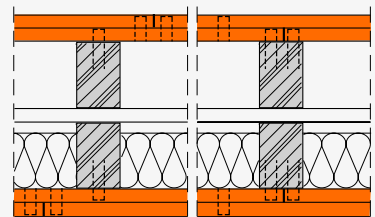
Montagewand mit fermacell® Gipsfaserplatten mit Hohlraumdämmung als Doppelständerwand, doppelagig bekleidet
