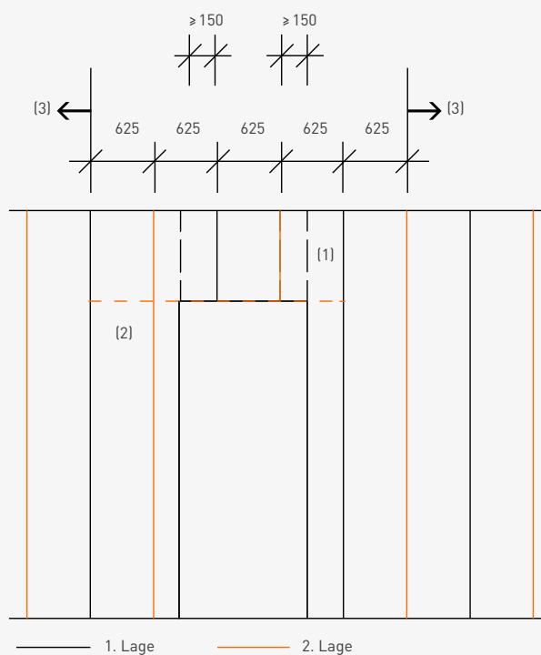
Bekleidung der Rückseite (Maße in mm)
