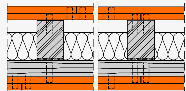
Montagewand mit fermacell® Gipsfaserplatten mit Hohlraumdämmung als Einfachständerwand mit Querhölzern, doppelagig bekleidet
