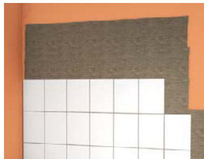
Abb. 9: Verfliesung mit fermacell™ Flexkleber im Dünnbettverfahren auf vollflächiger Abdichtung
