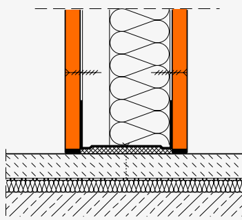
Trennwand auf durchlaufendem schwimmendem Estrich ( R_{L,w,R} ) = 38 dB*
