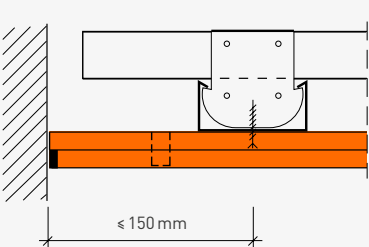
Anschluss mit elastischem Versiegelungsmaterial
