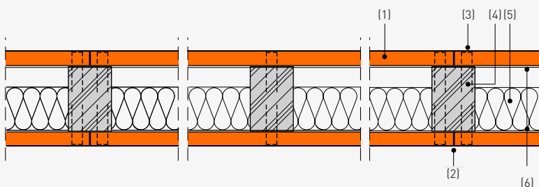
Montagewand mit fermacell® Gipsfaserplatten mit Stahl-/Holzunterkonstruktion
