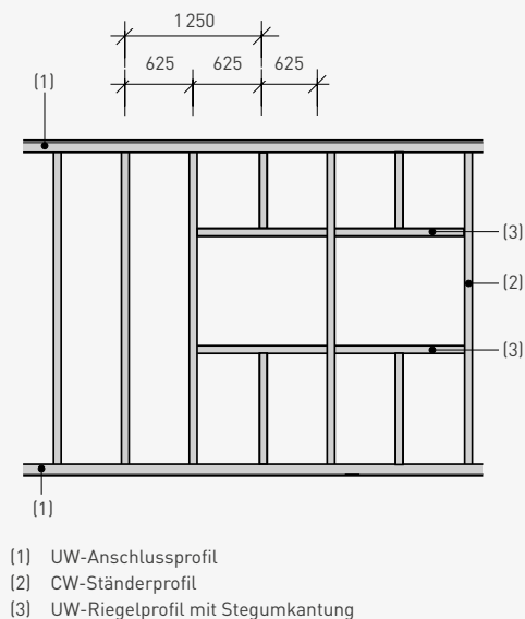
Ausbildung von Glasfeldöffnungen in der Montagewand mit fermacell® Gipsfaserplatten (Maße in mm)
