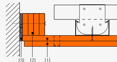
Anschluss mit Streifenbündel
