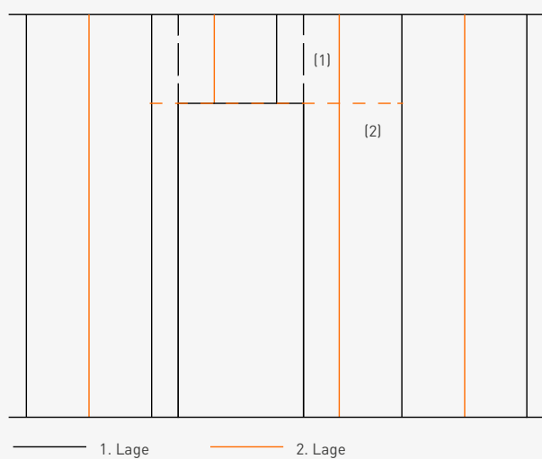
Bekleidungsschema zweilagig bekleidete Montagewand mit fermacell® Gipsfaserplatten
