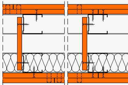
Verlascung bei einer Installationswand mit fermacell® Gipsfaserplatten
