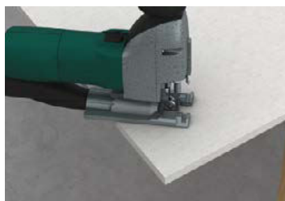
Sägen mit elektrischer Stichsäge
