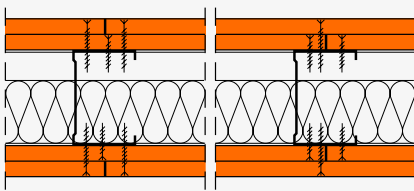
Montagewand mit fermacell® Gipsfaserplatten als Einfachständerwand, doppellagig bekleidet. Beide Plattenlagen in Ständerprofile verschraubt
