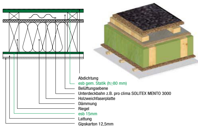
Abbildung 2 – Voldämmung mit unterlüfteter Dachhaut
