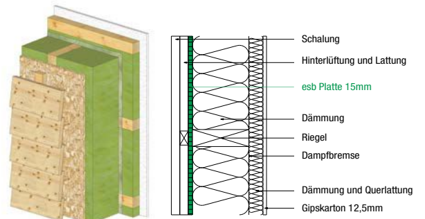
Außenwand 2 – hinterlüftet
