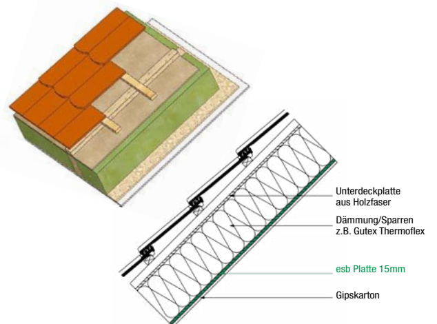
Dach 2 – Unterdeckplatte aus Holzfaser ohne aussteifende Wirkung
