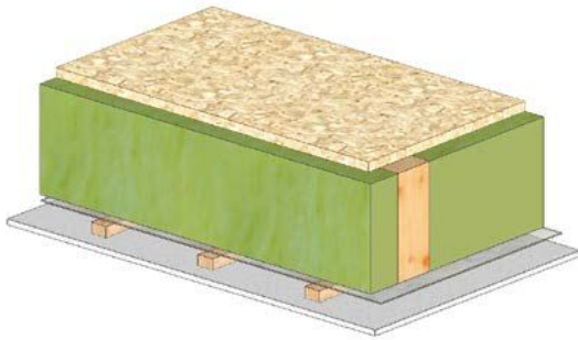
Innendecke 1 – zum unbeheizten Raum ESB-TIPP!
