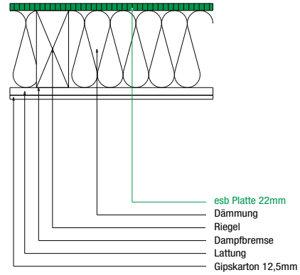
Innendecke 1 – zum unbeheizten Raum ESB-TIPP!
