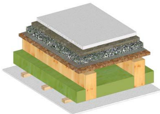
Innendecke 3 – zum beheizten Raum
