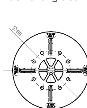
TERRASYS Schienengleiter
