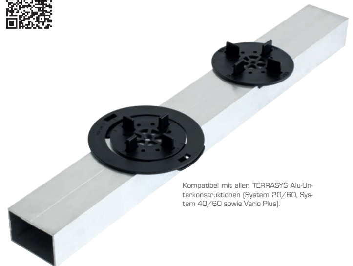
TERRASYS Schienengleiter
