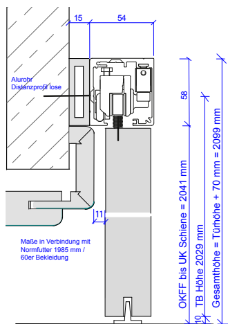
Wandmontage, mit Futter
