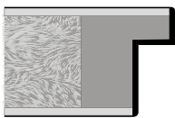
Türblatt Premiumkante (PK2)
