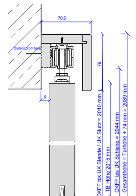
Außenlaufend, ohne Futter
