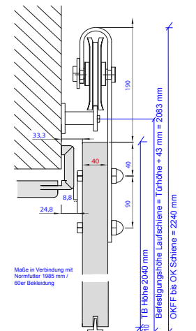
Außenlaufend, mit Futter
