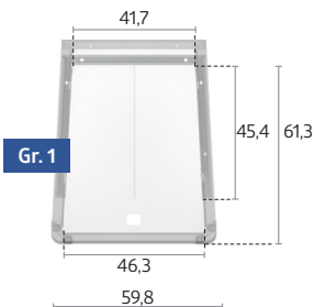
Draufsicht
