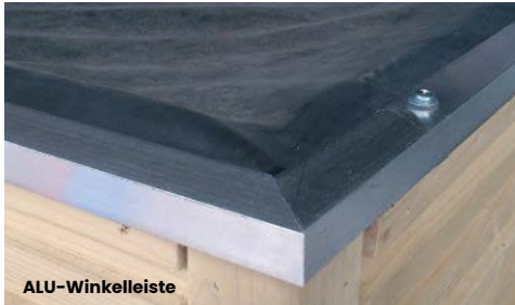
ALU-Winkelleiste
